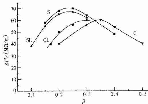
图 1 SDTL 和 CCDTL 的有效分路阻抗
