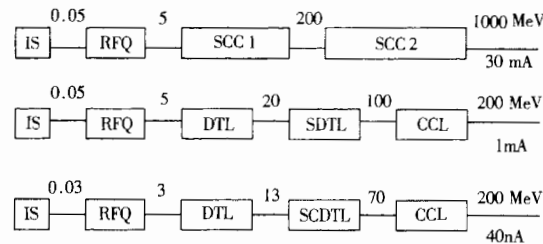
图 2 洁净核能系统连续束强流质子直线加速器(上)、L 波段多用脉冲束强流质子直线加速器(中)和 S 波段质子治疗直线加速器(下)
