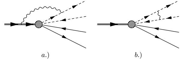
Fig. 7. example vertex diagrams [14].
