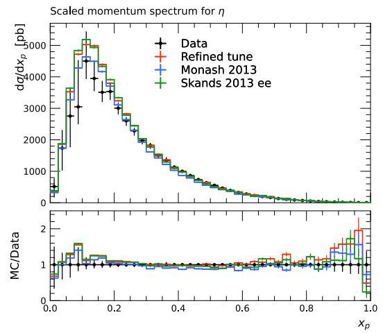
(d) \eta scaled-momentum spectrum.
