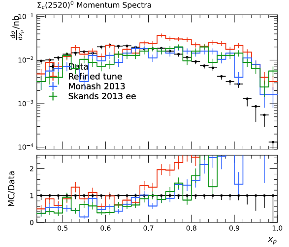
(d) \Sigma_c(2520)^0 momentum spectrum.
